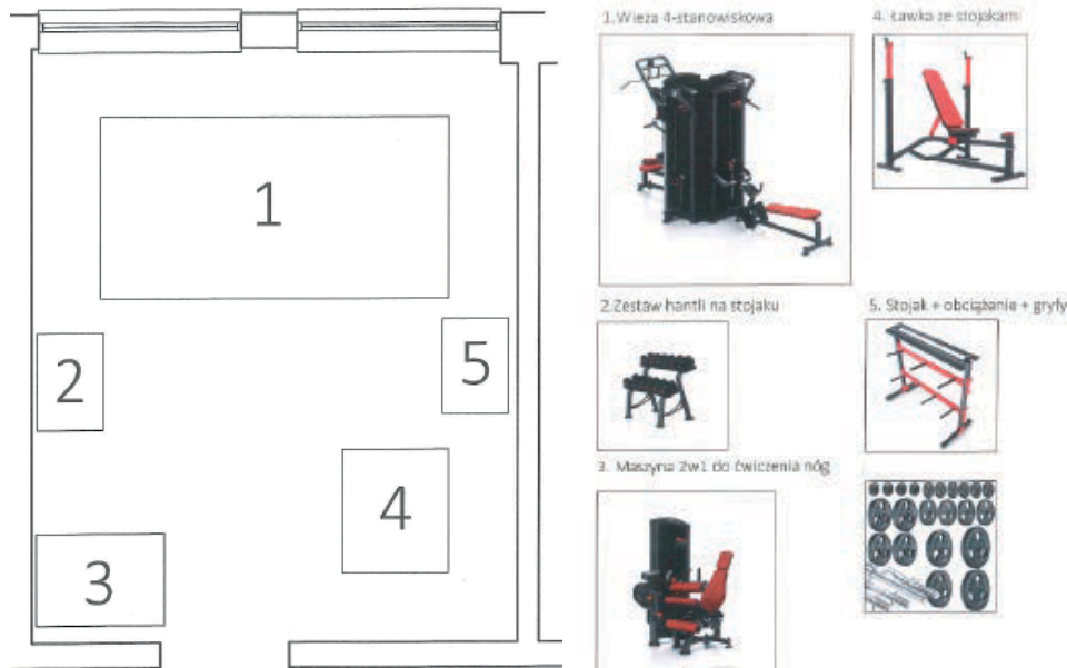
Wizualizacja siłowni
